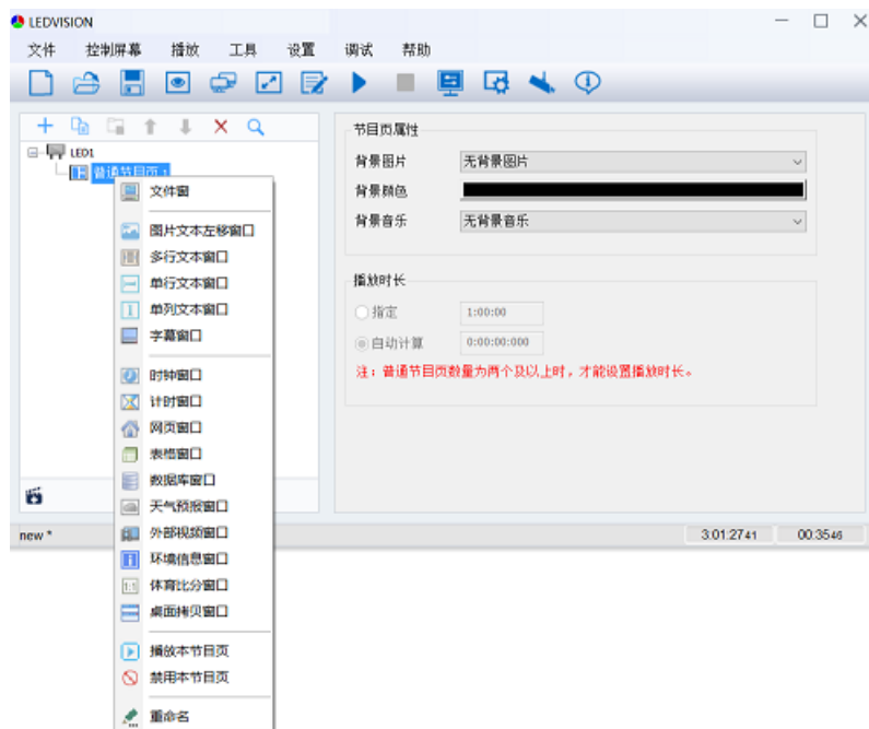
图 4-9 添加节目窗口
