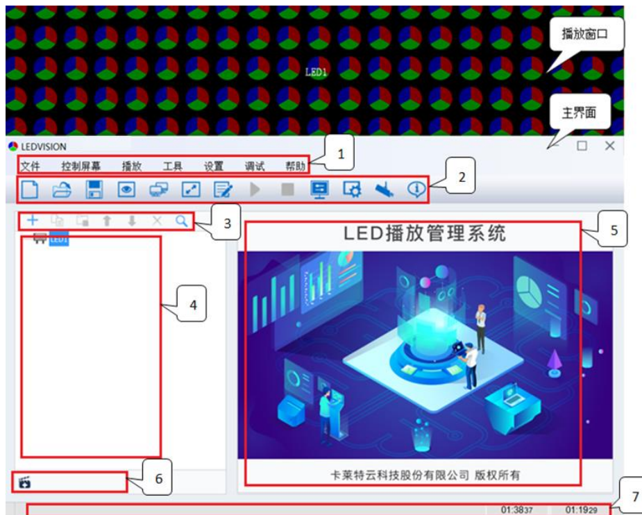
图 3-1 LEDVISION 软件主界面
