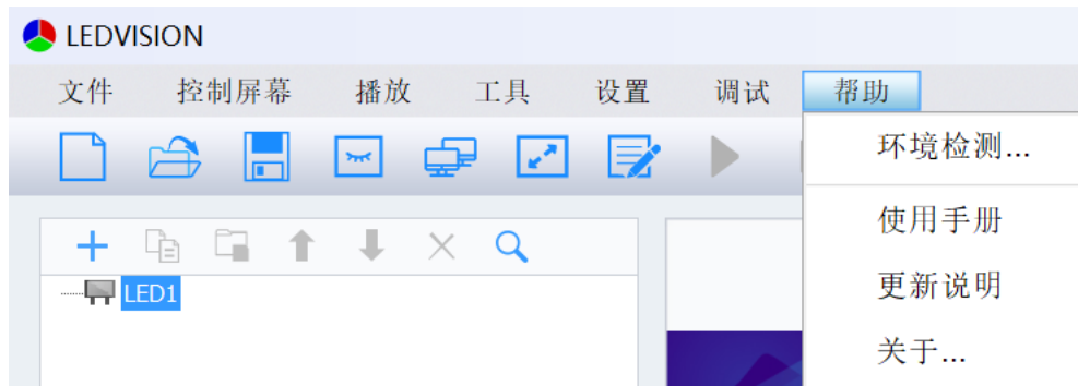
图 3-9 帮助菜单
