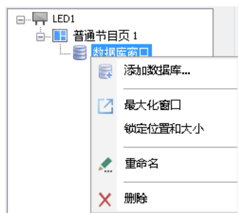
图 5-30 新建数据库
