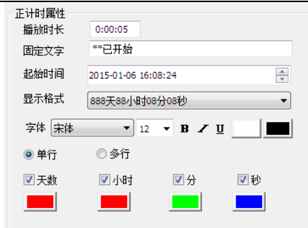
图 5-23 计时属性
