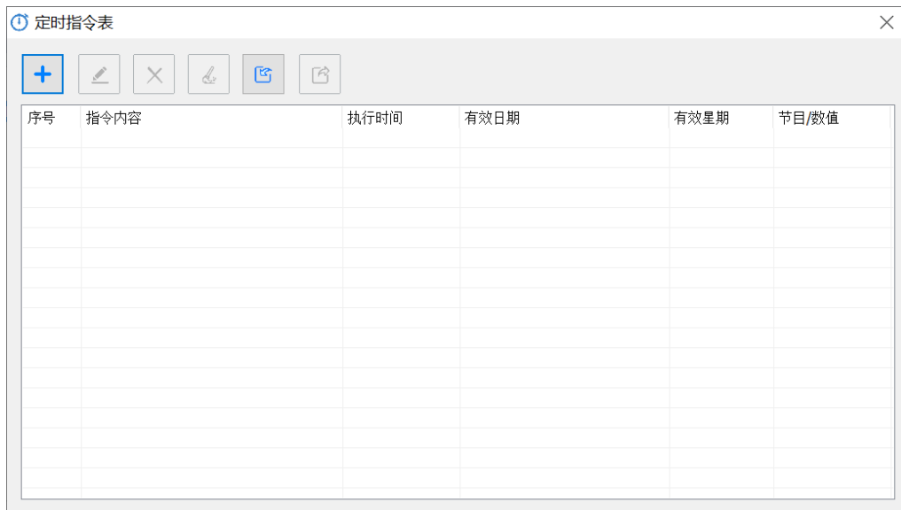
图 7-1 定时指令表
