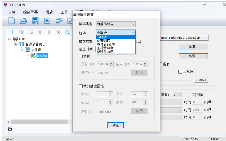
图 8-7 视频旋转
