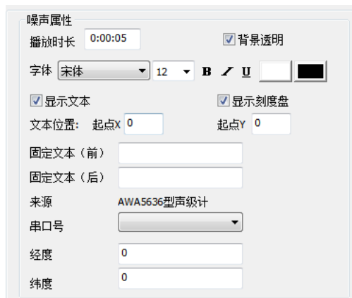
图 5-55 噪音属性
