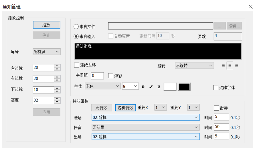
图 6-1 通知管理
