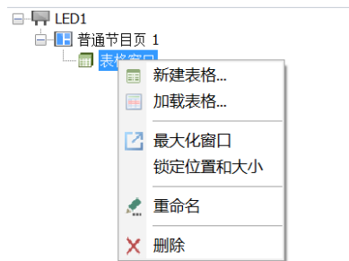
图 5-28 新建表格
