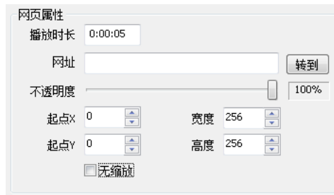
图 5-27 网页缩放
