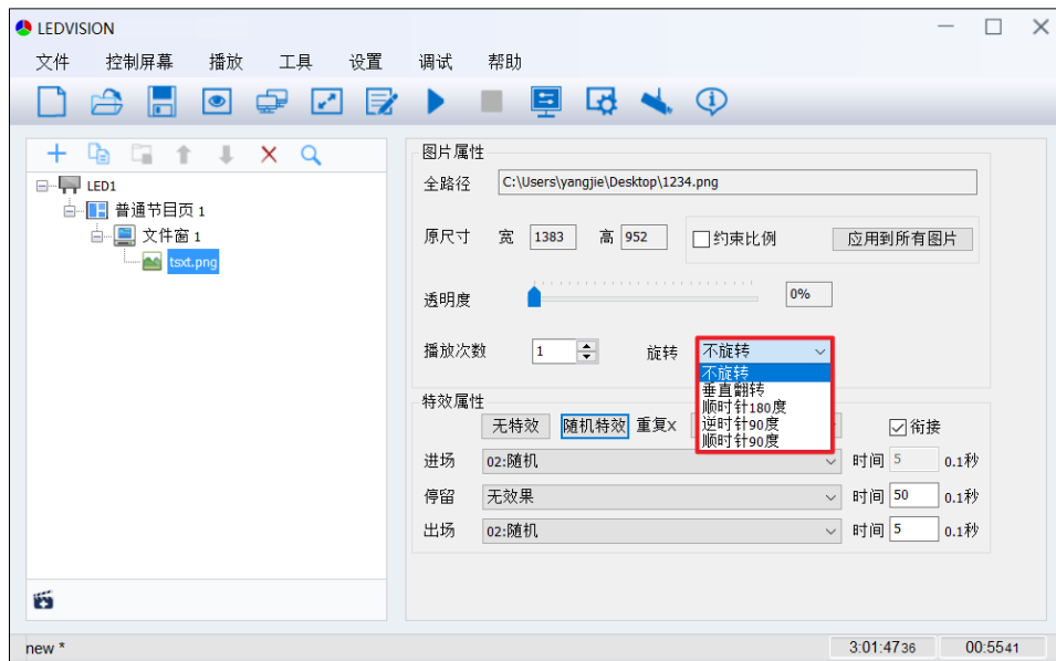
图 8-6 图片旋转
