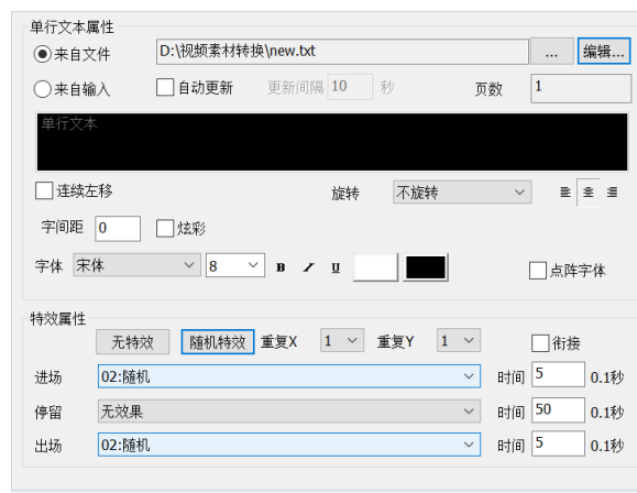
图 5-14 单行文本属性
