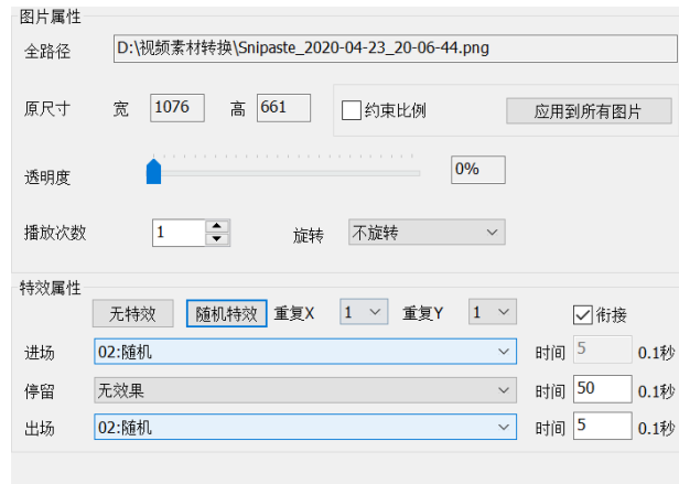
图 5-4 图片属性
