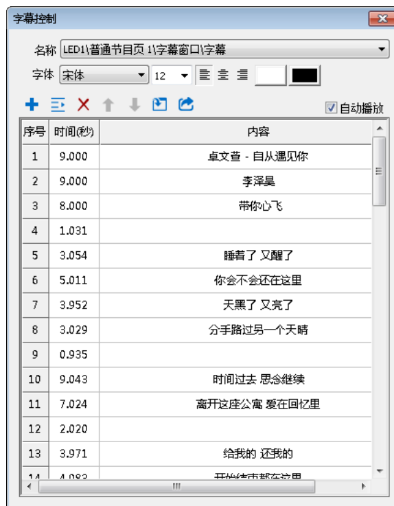
图 5-19 字幕控制
