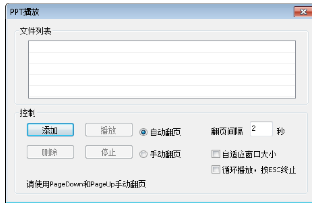
图 6-3 PPT 播放
