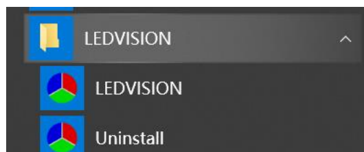
图 2-6 卸载 LEDVISION
