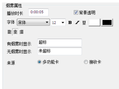
图 5-54 烟雾属性
