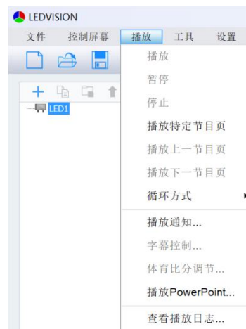
图 3-5 播放菜单
