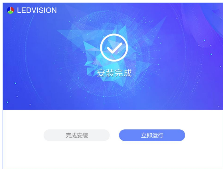
图 2-5 安装完成
