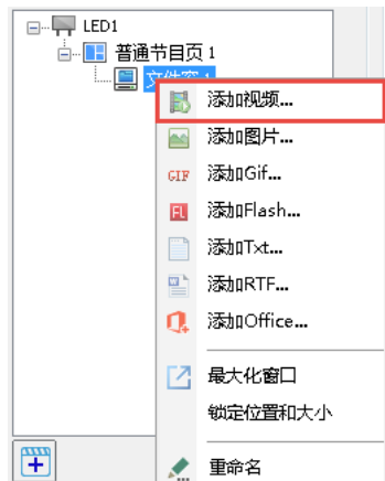
图 5-1 添加视频
