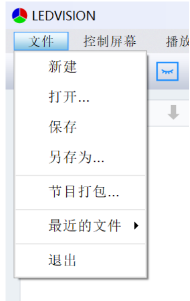
图 3-3 文件菜单栏
