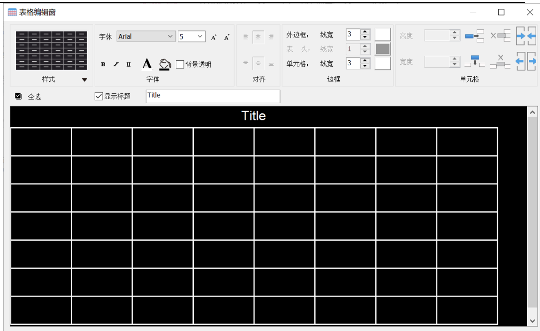
图 5-29 表格编辑窗
