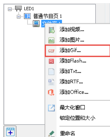
图 5-5 添加 Gif
