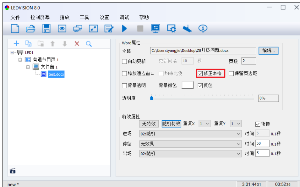
图 8-4 修正表格
