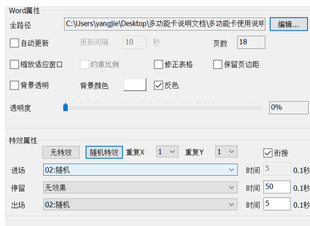
图 5-9 Word 属性
