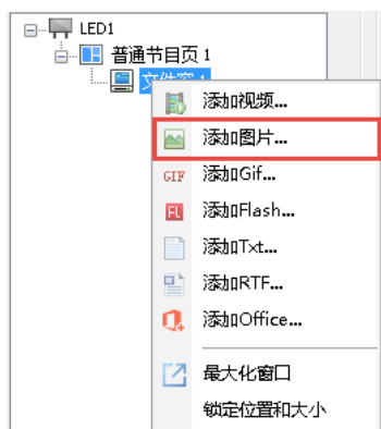
图 5-3 添加图片
