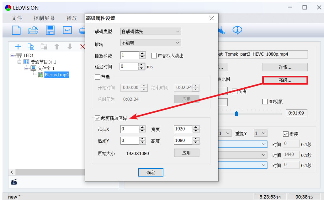
图 8-1 视频裁剪
