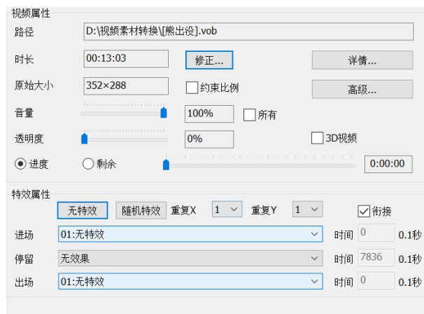
图 5-2 视频属性
